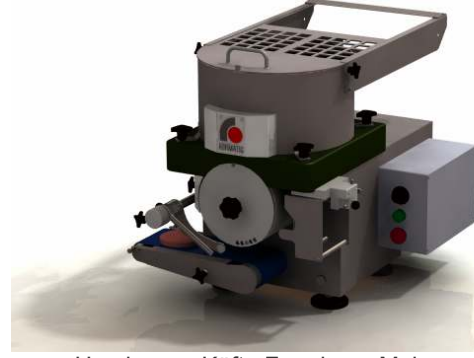
Hamburger Köfte Formlama Mak. 2200 – 8000 vuruő / saat
